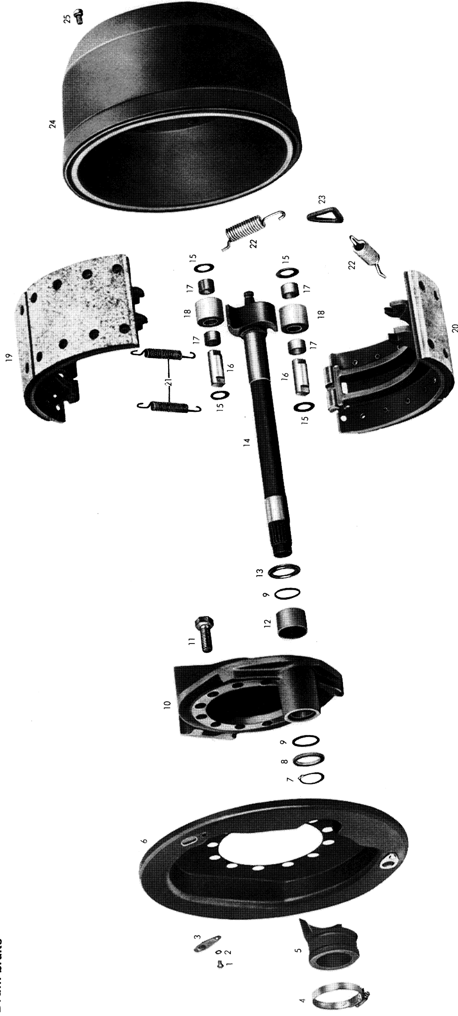
Tafel/Table 6 Trommelbremse Drum brake
