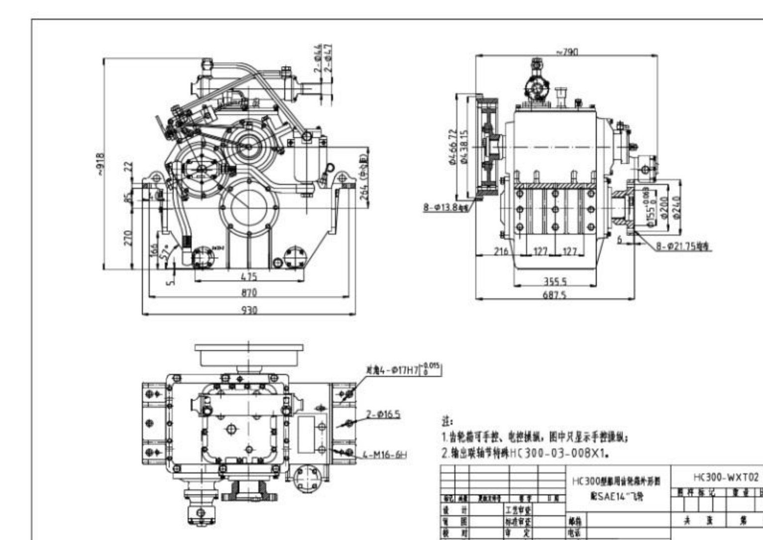
输出联轴节特殊HC300-03-008X1
