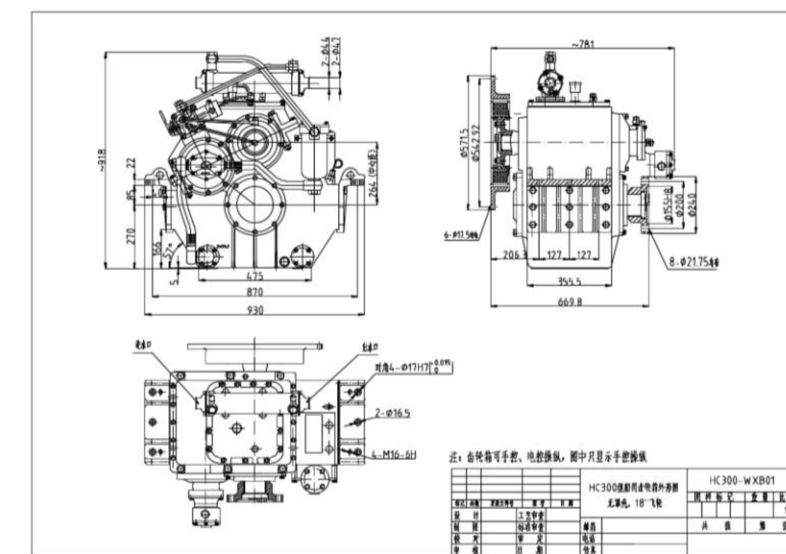
SAE18"高弹-WXB01
