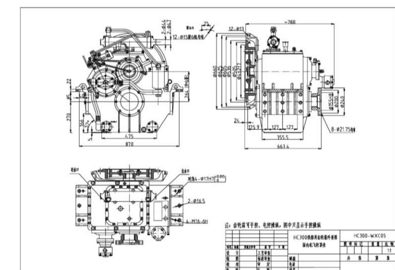
国内机罩壳齿形块-WXC05
