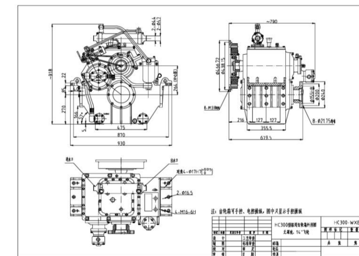
SAE14"高弹-WXB03
