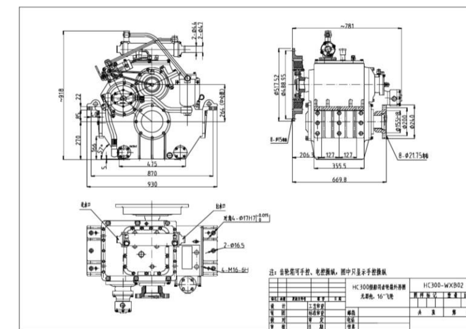
SAE16"高弹-WXB02
