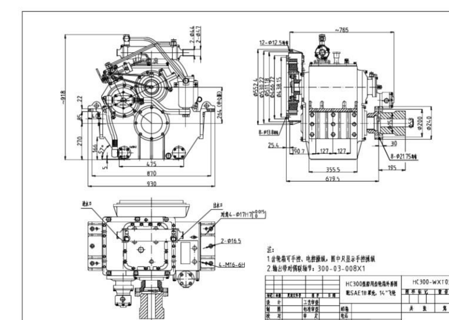
输出带对偶联轴节: 300-03-008X1
