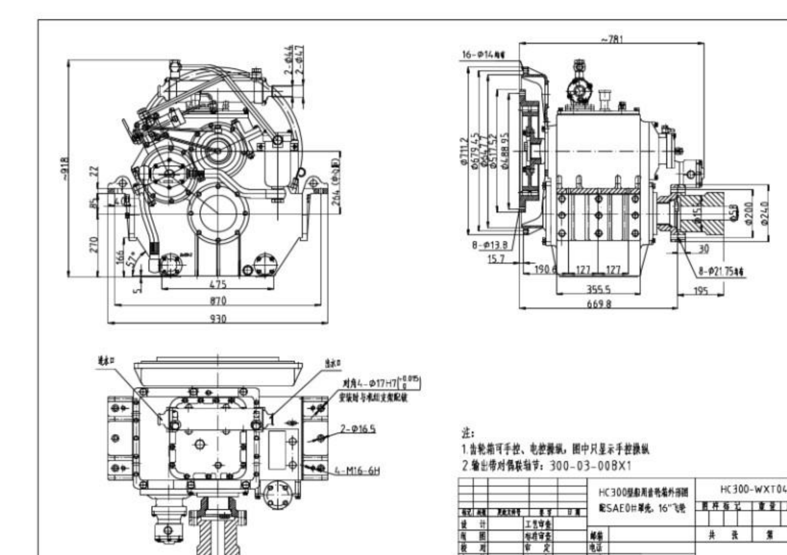
输出带对偶联轴节: 300-03-008X1
