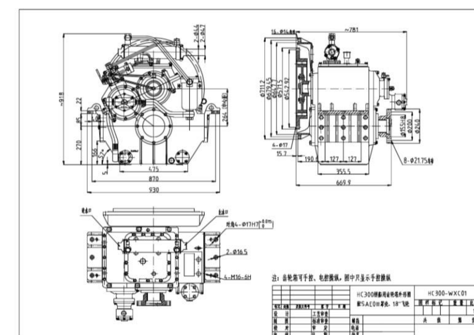
SAE0#罩壳 18"齿形块-WXC01
