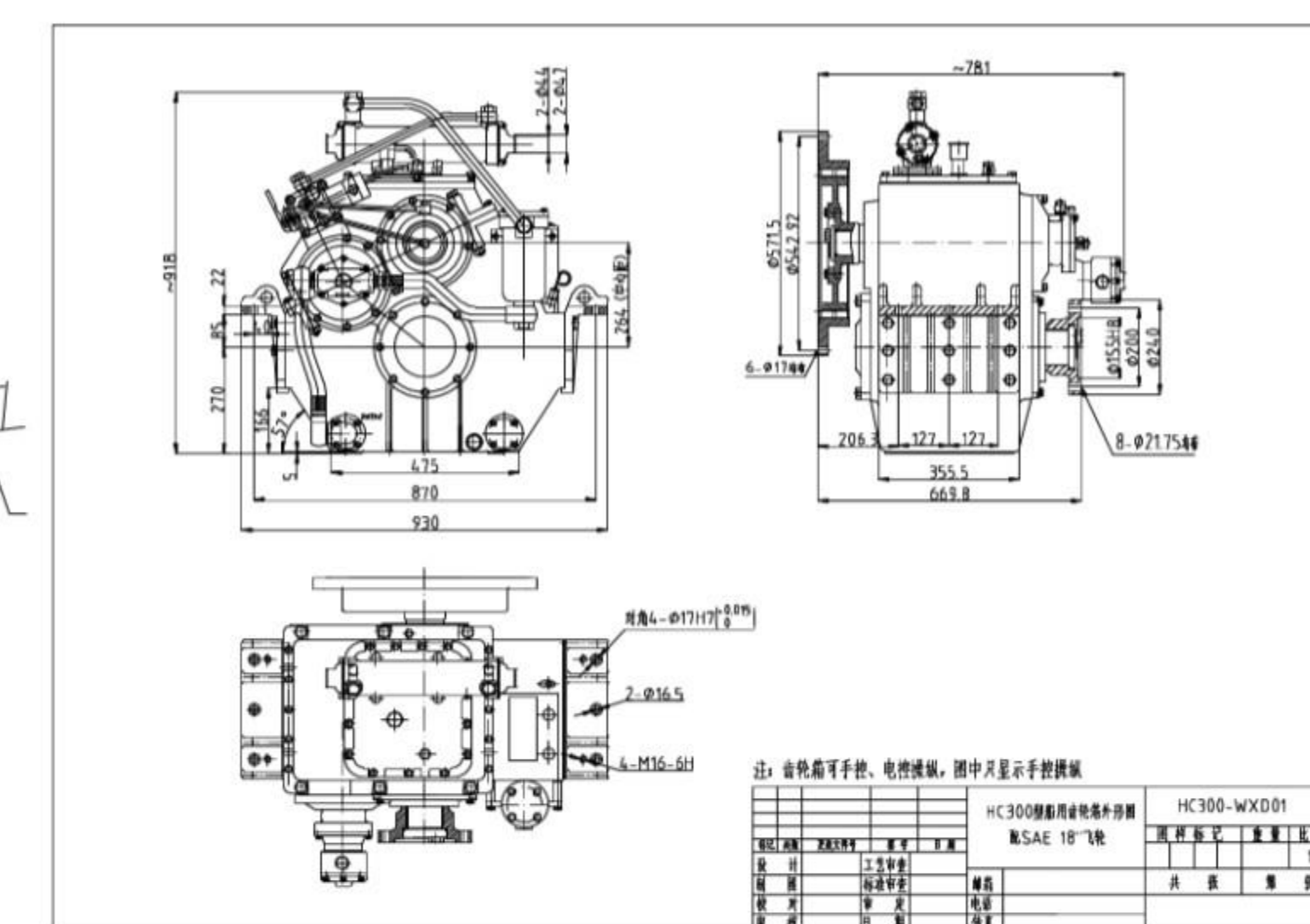
SAE18"齿形块-WXD01
