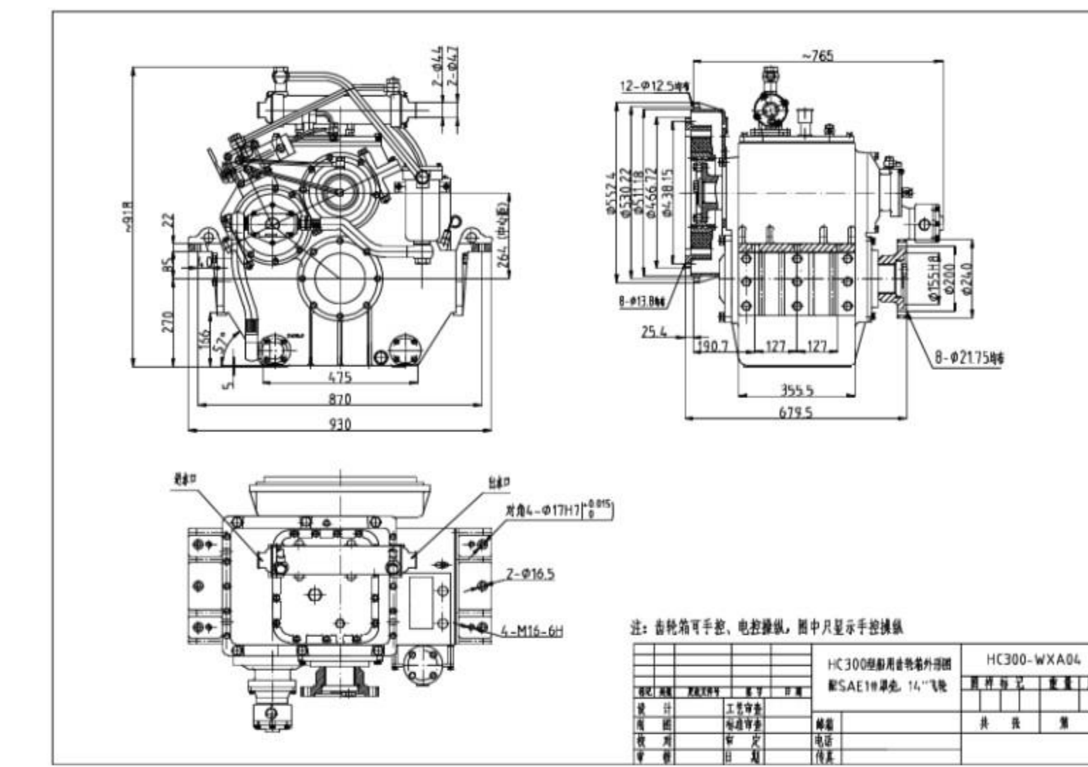
SAE1#罩壳 14"高弹-WXA04
