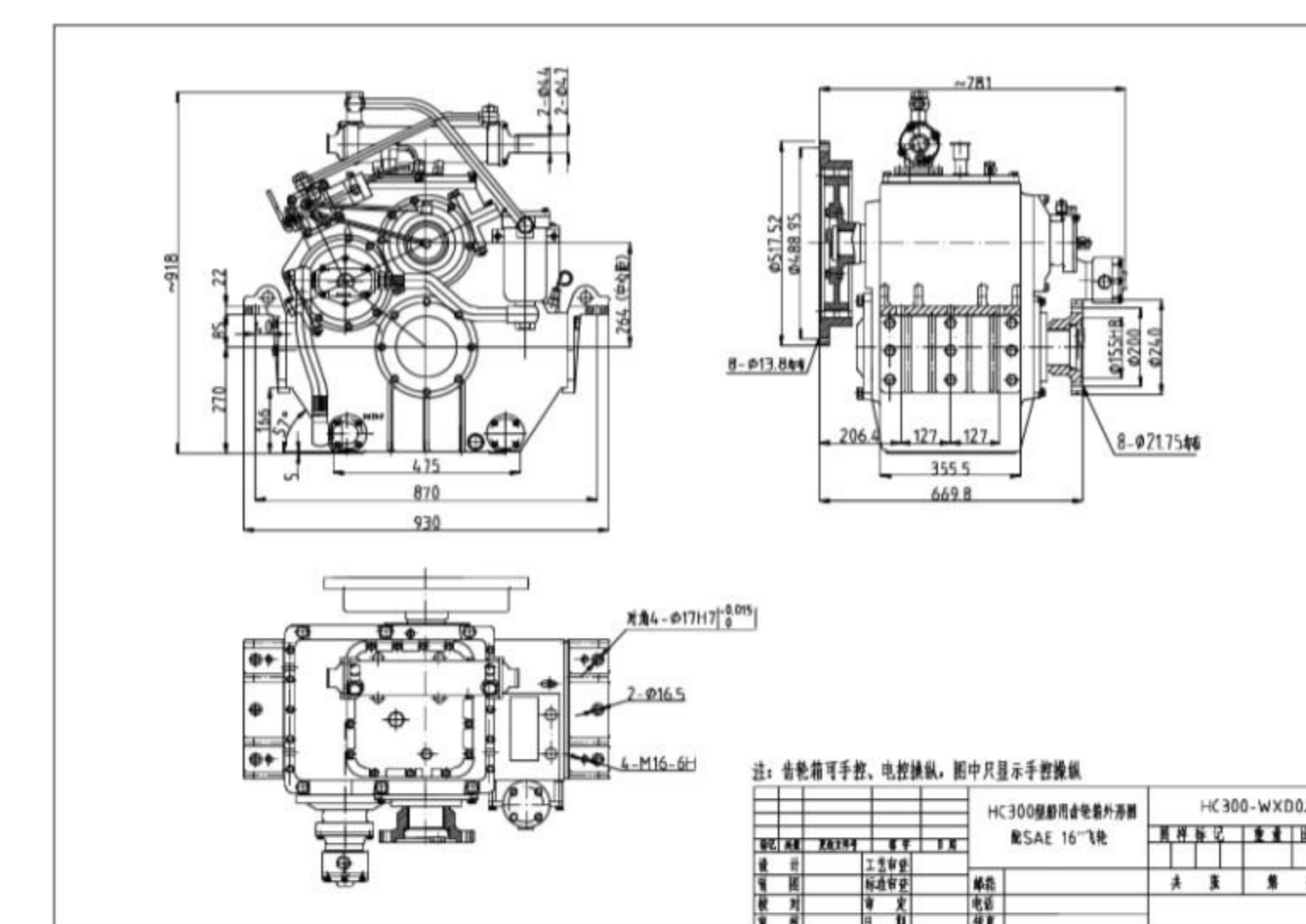
SAE16"齿形块-WXD02
