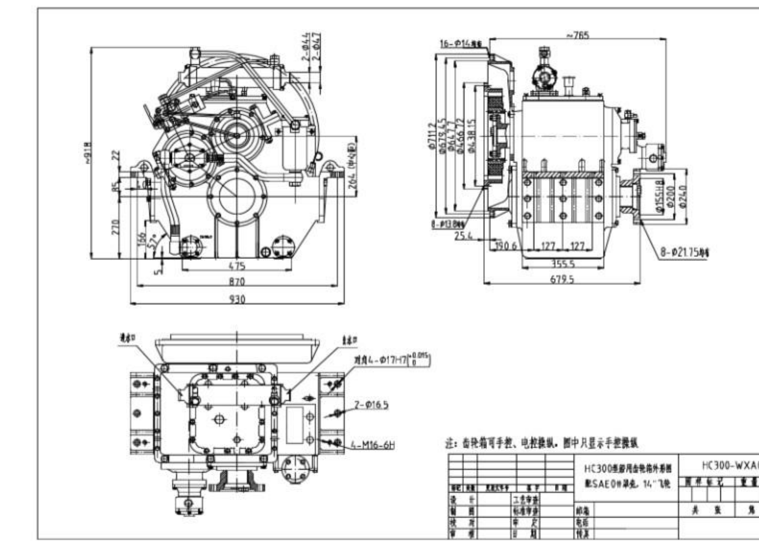
SAE0#罩壳 14"高弹-WXA03
