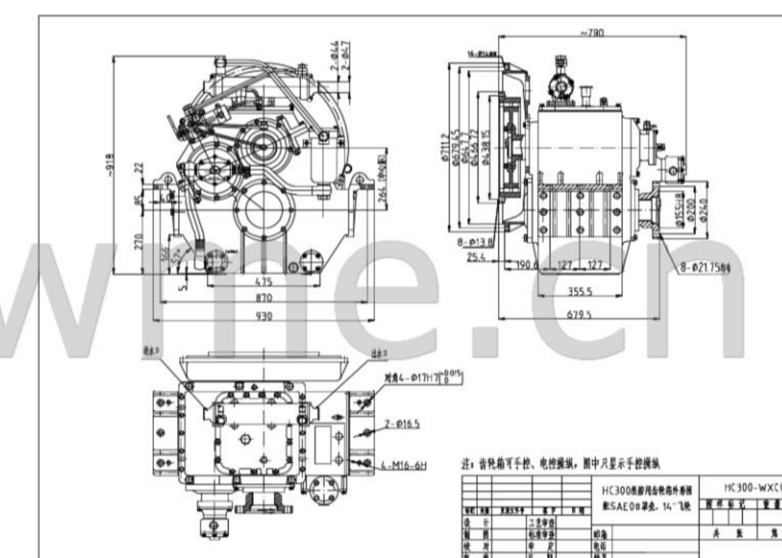
SAE0#罩壳 14"齿形块-WXC03
