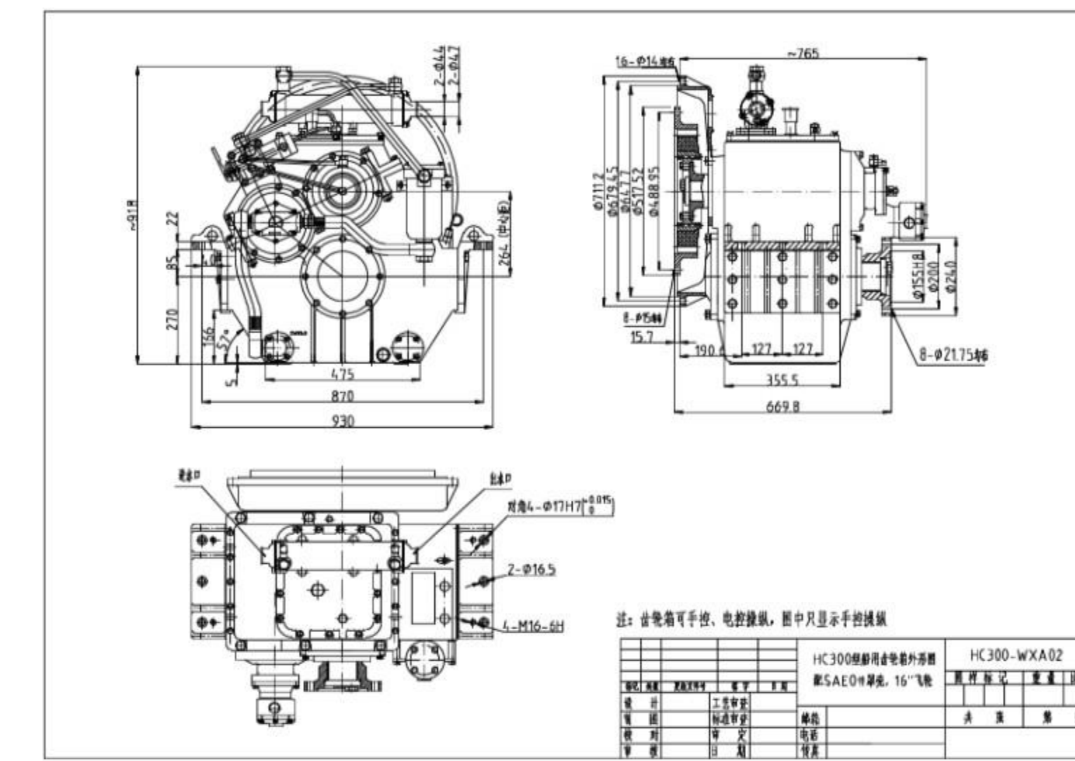
SAE0#罩壳 16"高弹-WXA02
