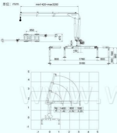
SQ1ZK2Q 起重机主要技术参数 MAIN SPECIFICATION
