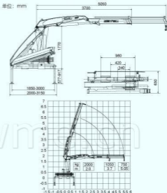
SQ2ZK1 起重机主要技术参数 MAIN SPECIFICATION
