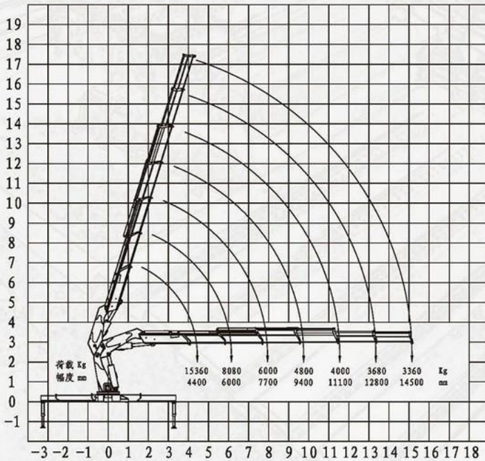
SQ500 ZB6 起升性能曲线
