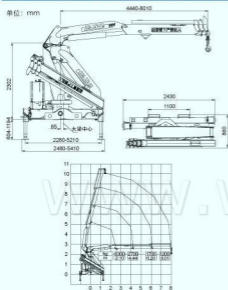
SQ6.3ZK2Q 起重机主要技术参数 MAIN SPECIFICATION
