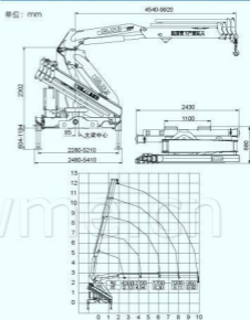
SQ6.3ZK3Q 起重机主要技术参数 MAIN SPECIFICATION
