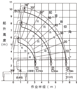
URV343起重特性曲线
