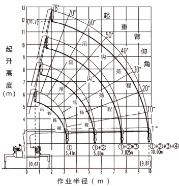
URV344起重特性曲线
