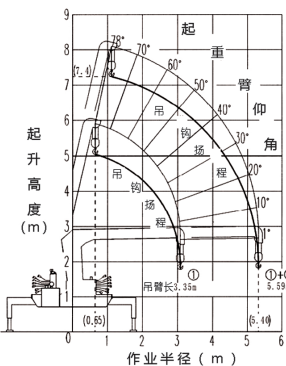
URV342起重特性曲线
