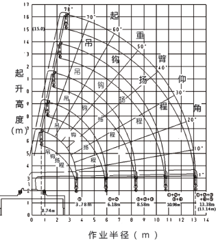
URV505起重特性曲线
