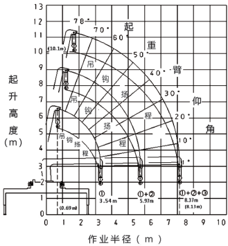
URV503起重特性曲线
