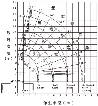
URV504起重特性曲线
