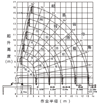
URV635起重特性曲线
