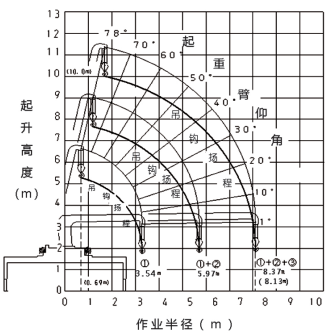
URV633起重特性曲线
