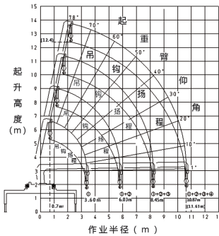
URV634起重特性曲线
