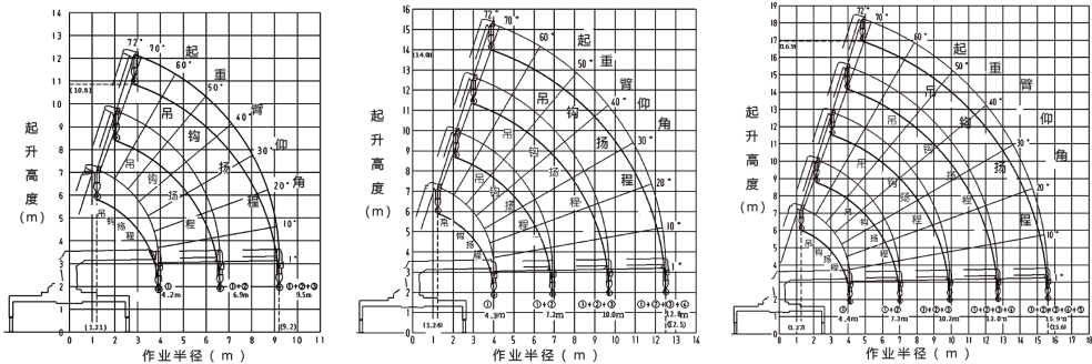
URV803起重特性曲线
