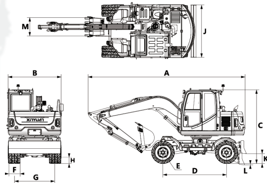
★外形尺寸图
