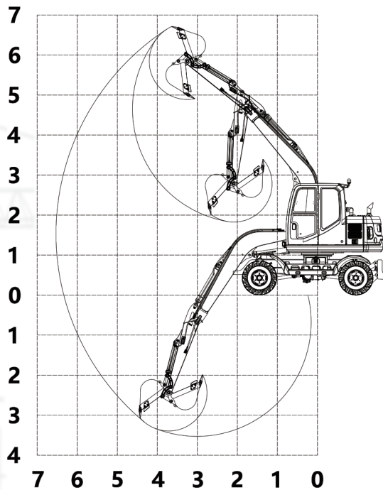
★作业范围图
