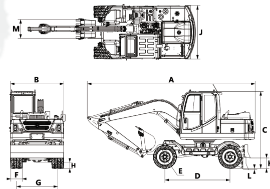
★外径尺寸图
