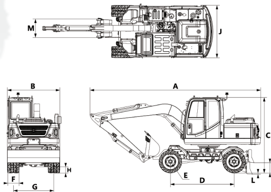
★外形尺寸图
