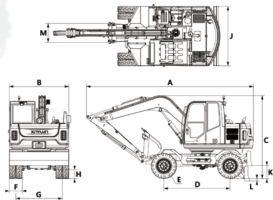
★外形尺寸图
