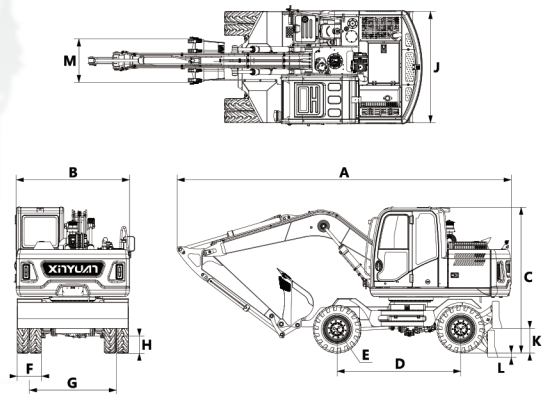
★外形尺寸图
