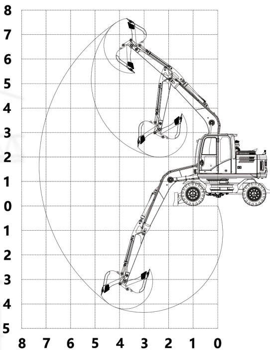
★外形尺寸图
