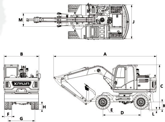
★外形尺寸图
