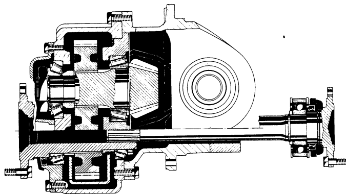
Achseinsatz DK - 7 Differential carrier DK - 7
