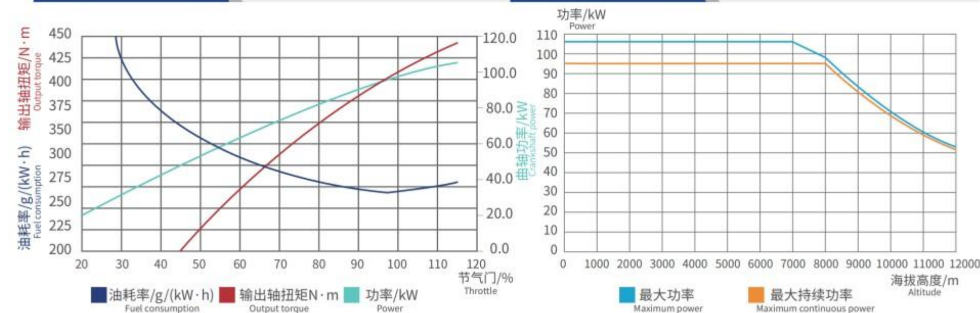
负荷特性曲线
